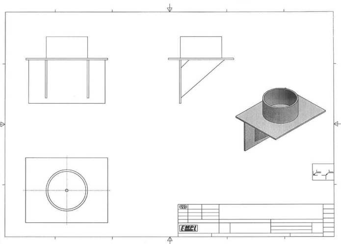
Übungswerkstück Autogenschweißen
